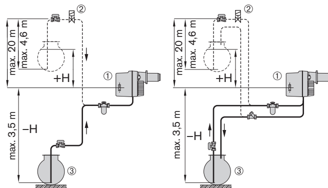
Système mono-tube
