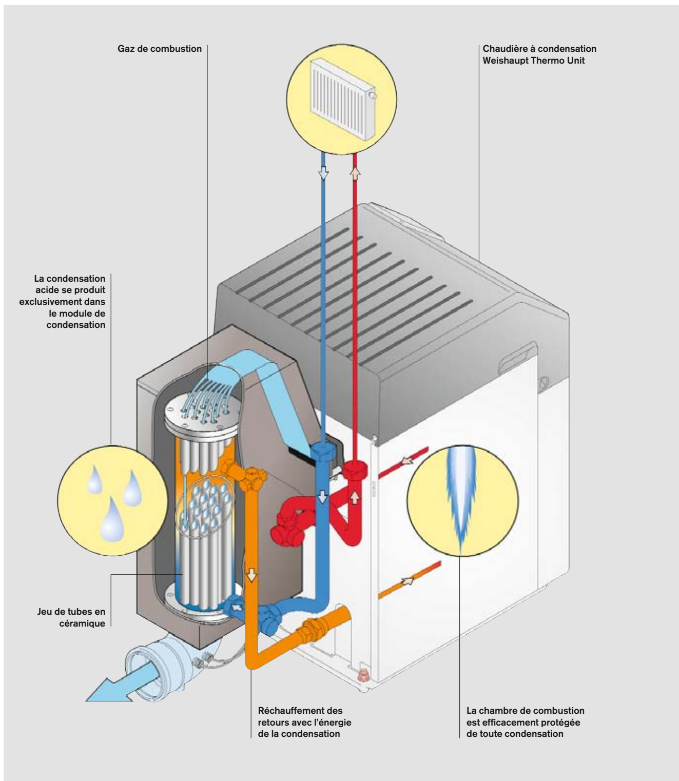
Le principe de condensation fioul Weishaupt
