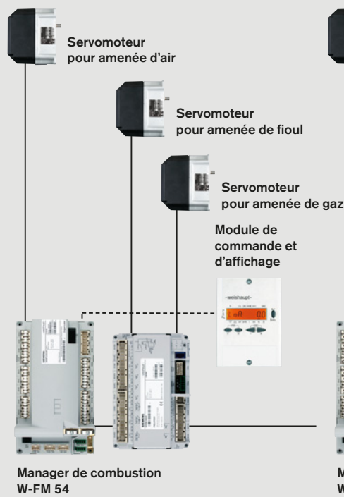
Schéma de principe du W-FM 54
